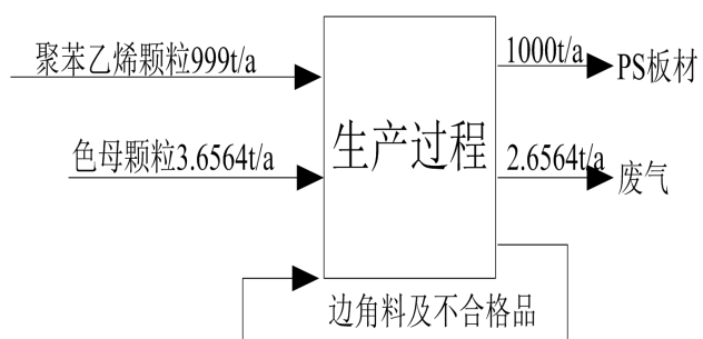
图2-1 本项目物料平衡图
