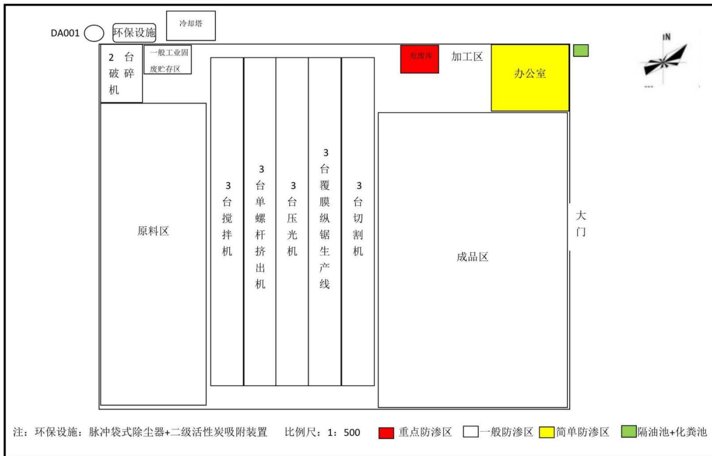
附图三 厂区平面布局图
