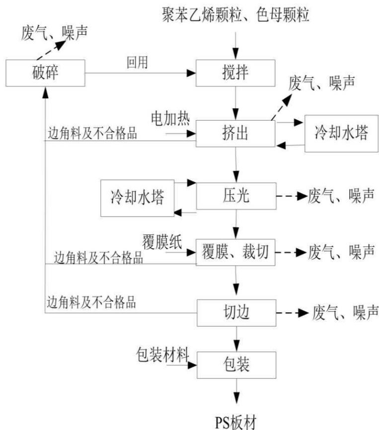
图1 生产工艺流程及产污环节示意图
