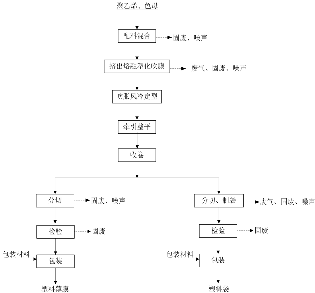
图 2-3 项目工艺流程及产污环节示意图
