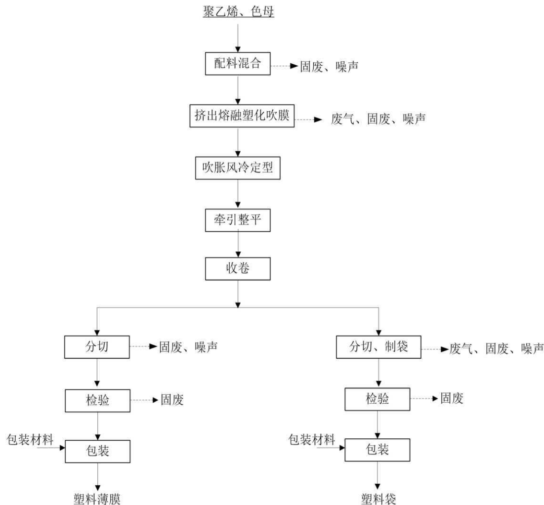
图 1 项目工艺流程及产污环节示意图
