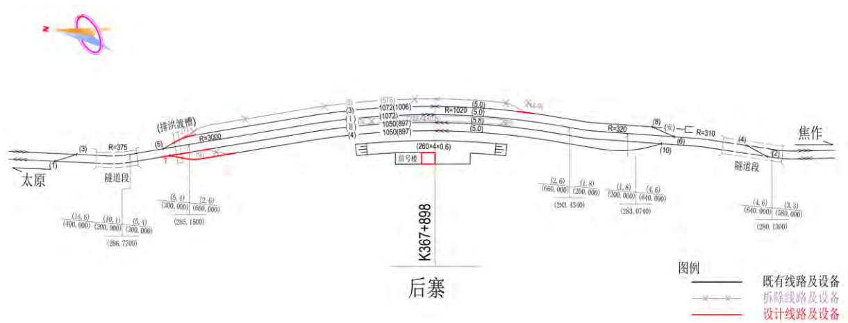
图 2-1 后寨站改造方案示意图
