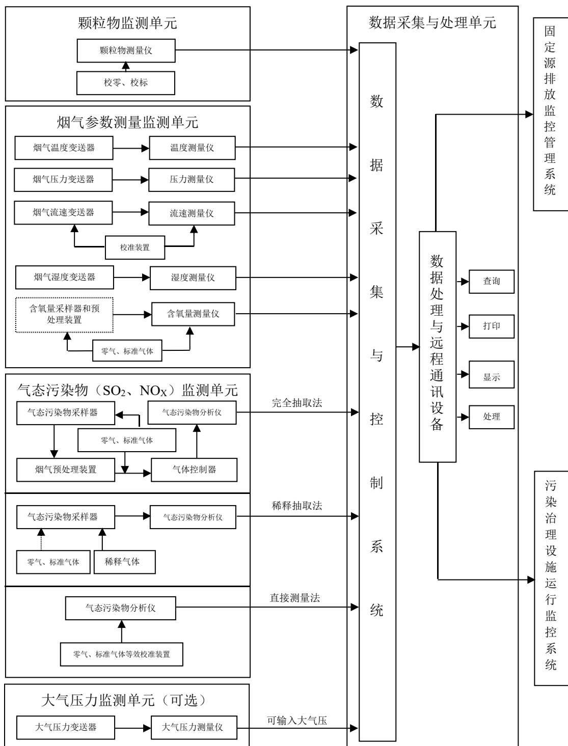
图 1 固定污染源烟气 (SO 2 、NO x 、颗粒物) 排放连续监测系统组成示意图
