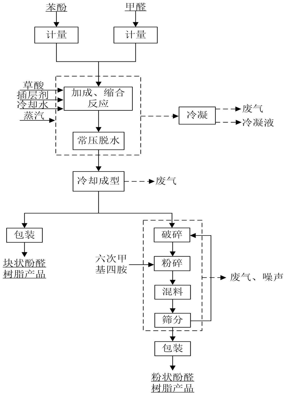
图 4.1-2 固态酚醛树脂产品生产工艺及产污环节流程图
