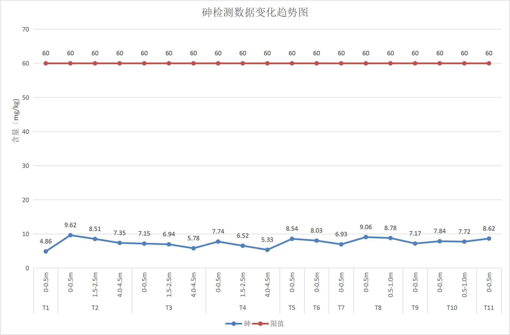
图 8-1 砷检测数据变化趋势图
