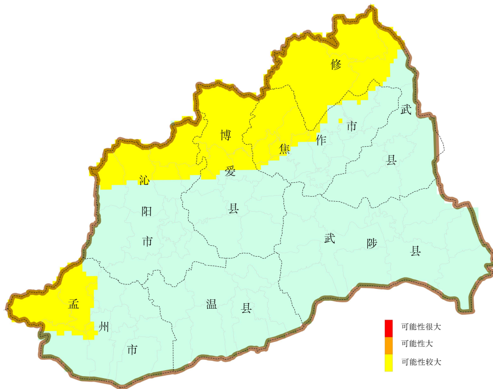
图 2 焦作市汛期地质灾害气象风险预警成果图
